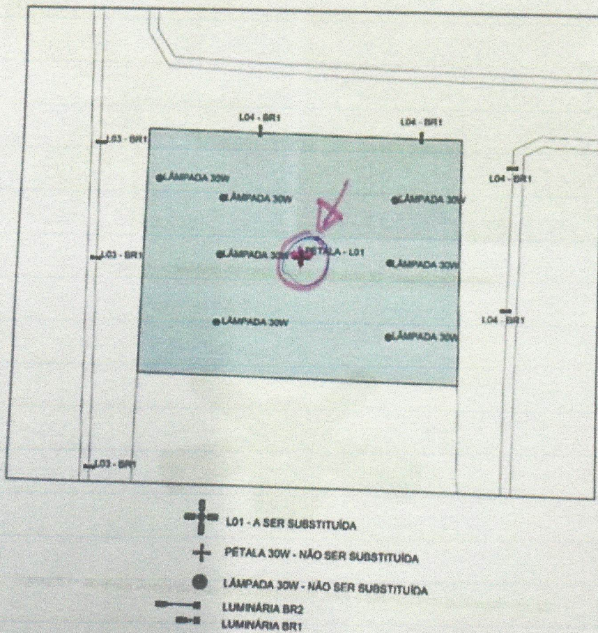
Figura 3 — Diagrama esquemático da distribuição das luminárias na praça Pedro Álvares Cabral e marcação da luminária que será substituída.
